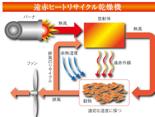
ヒートリサイクル制御の概要
